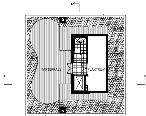
PLAN 6, GEMENSAMT UTERUM OCH TAKTERRASS
