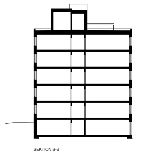
SEKTION B-B
