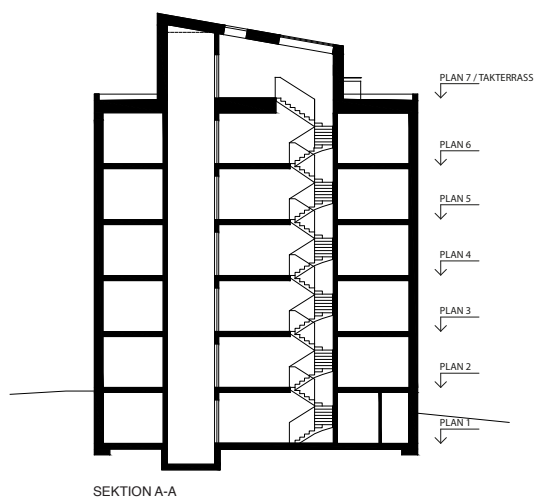
SEKTION A-A
